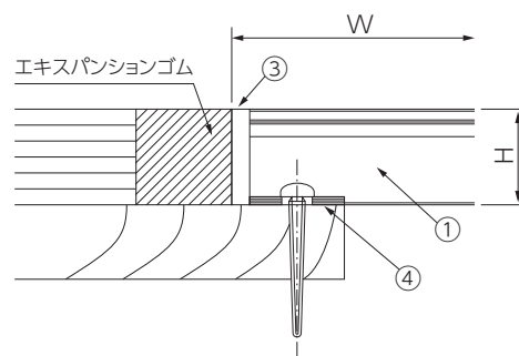
■納まり図
